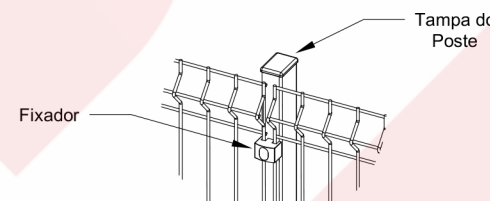
Det. B esc. 1:10
