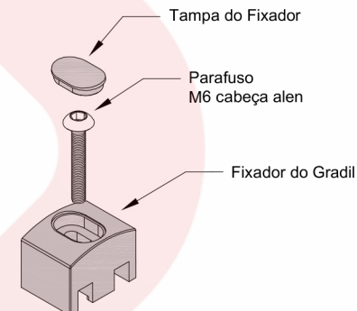
Tampa do Fixador
