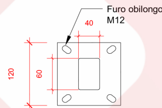
Detalhe A Base Poste esc. 1:5
