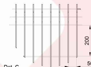
Det. C esc. 1:10
