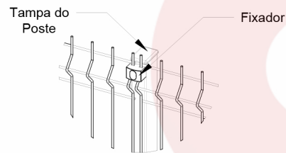
Det. B esc. 1:10
