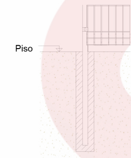
Detalhe A Base Poste esc. 1:20
