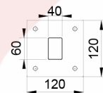
Detalhe A Base Poste esc. 1:10
