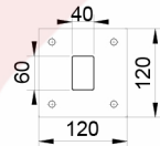
Detalhe A Base Poste esc. 1:10
