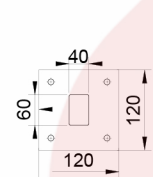
Detalhe A Base Poste esc. 1:10
