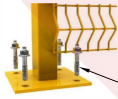
Detalhe A Base Poste esc. 1:10
