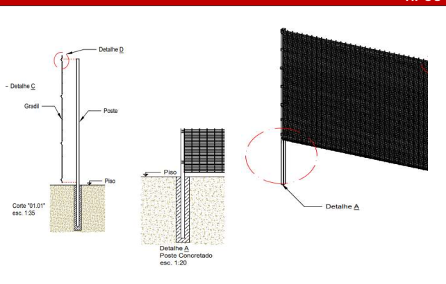
BASE CONCRETADA
