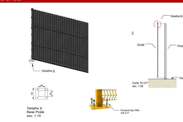
BASE APARAFUSADA
